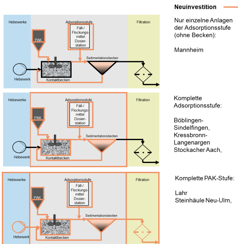
Abbildung 2: Unterschiedlicher Umfang der Neuinvestitionen (orange markierte Anlagenstufen) – entscheidend für Investitionskosten und historische Kapitalkosten
