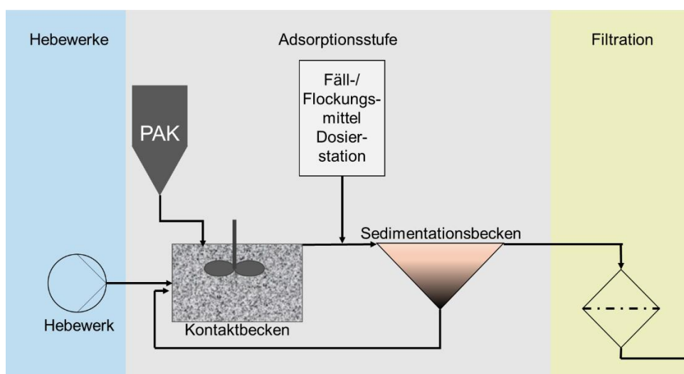
Abbildung 1: Betrachtete Anlagenteile in der PAK-Stufe
